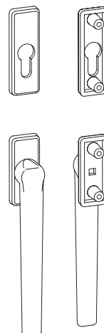
12 Manilla exterior 161 EG-PzA para cremón e/ bombillo
