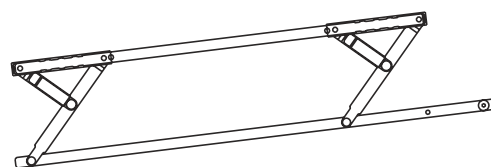
26 Grupo tijeras
