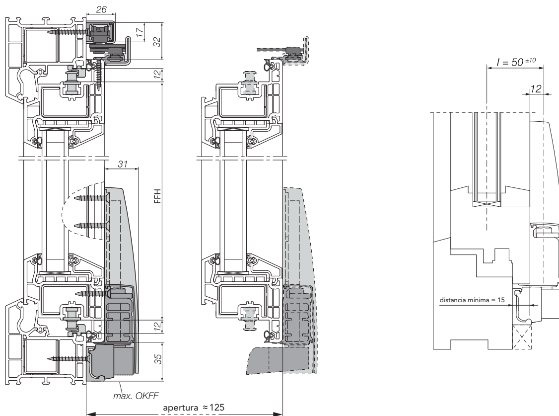
Sección vertical PVC
