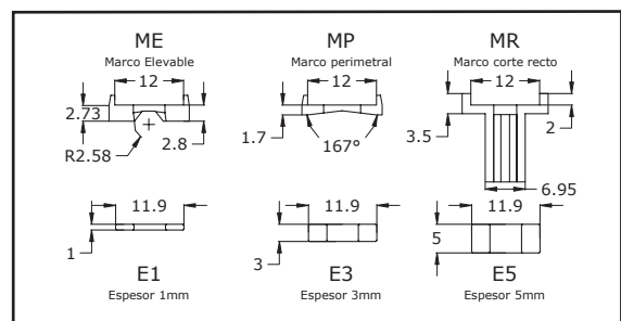
Calzos de cerradero *
