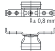
BISAGRA PARA APERTURAS ABATIBLES | presión ajustable
