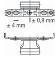
BISAGRA LATERAL SUPERPUESTA | presión ajustable y reg. aut. altura
