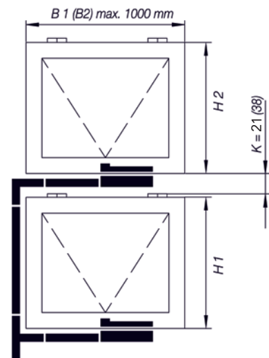
PRIMAT-A tipo f: 2 hojas superpuestas
