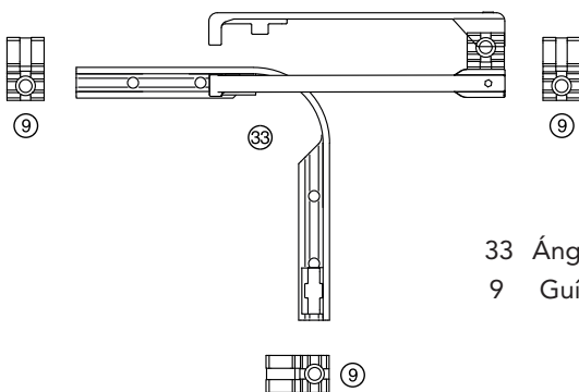
PRIMAT-A tipo hm: 2 hojas una al lado de otra
