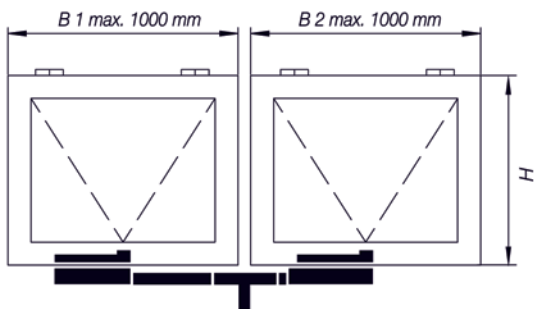
PRIMAT-A tipo hm: 2 hojas una al lado de otra
