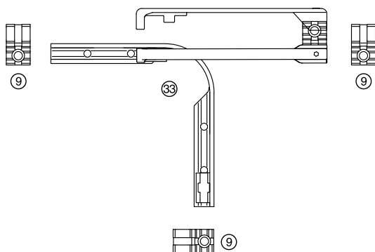
PRIMAT-FL 190, tipo hm: 2 hojas una al lado de otra
