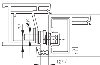
Sección vertical en PVC
