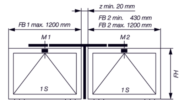
PRIMAT-FL 190, tipo hm: 2 hojas una al lado de otra
