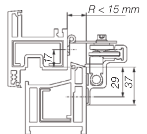
Sección vertical con soporte de tijera 2
